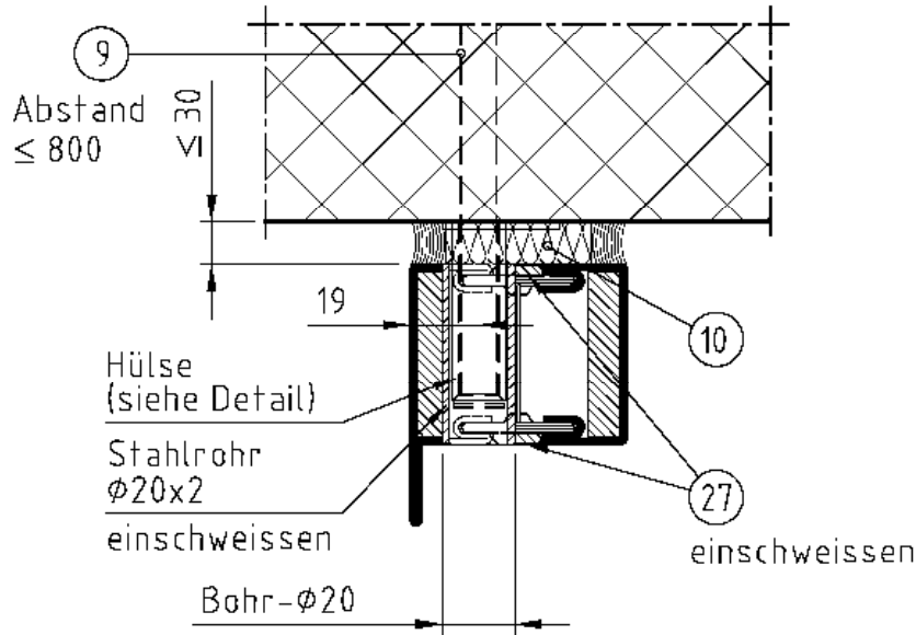
Detail Hülse für Teleskop-Deckenanschluss
