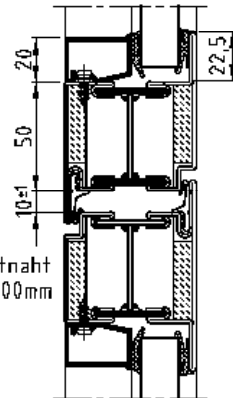
Schnitt F - F
