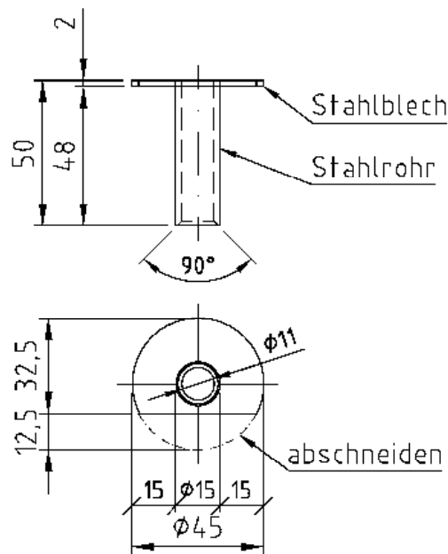
Detail Hülse für Teleskop-Deckenanschluss
